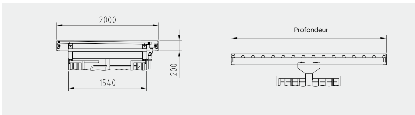
Toit D2 – avec cache en tôle trapézoïdale, profil de bandeau et écoulement
